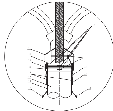
预制式电缆终端示意图
