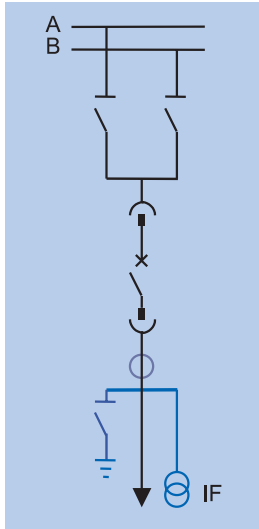
IF 进线/馈线单元
