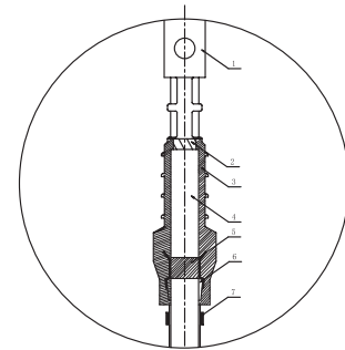
预制式电缆终端示意图
