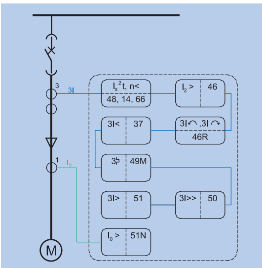
图六：典型基本要求电动机馈线保护
