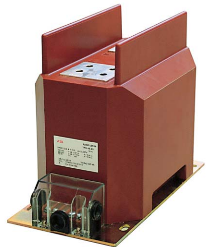
2500 A 电流互感器
