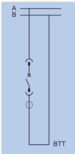
BTT 横向母联单元
